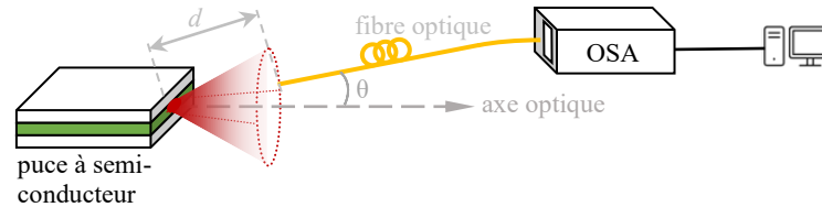
Fig. 1 : Schéma de principe du montage de caractérisation du champ lointain résolu spectralement.
